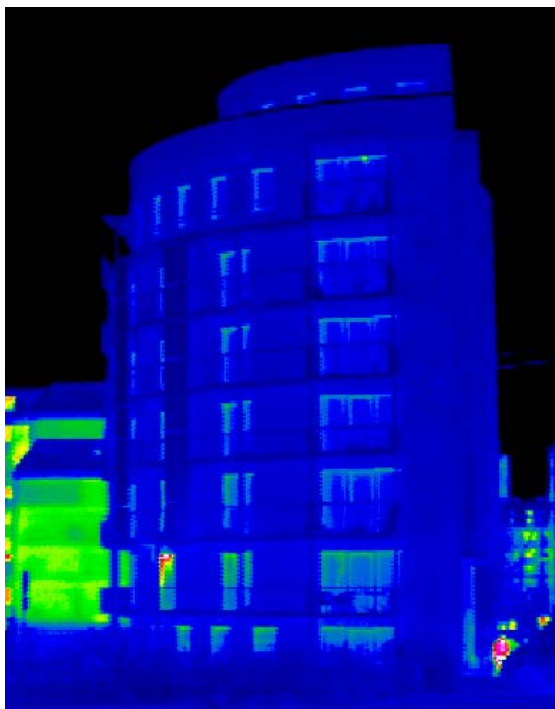
Passivhaus Pinnaasberg 27 am Hafenanrand: Traumhafter Blick und behagliches Raumklima. Thermografie mit Mensch und einem offenen Fenster
